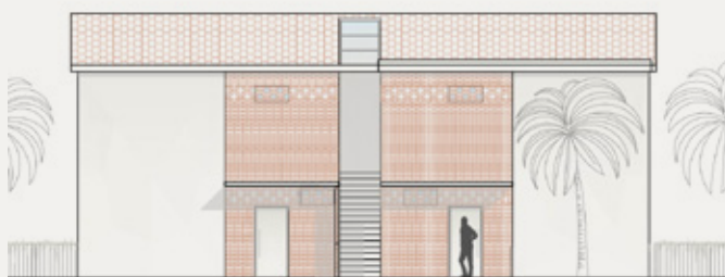
Ansicht Nord-Westen
